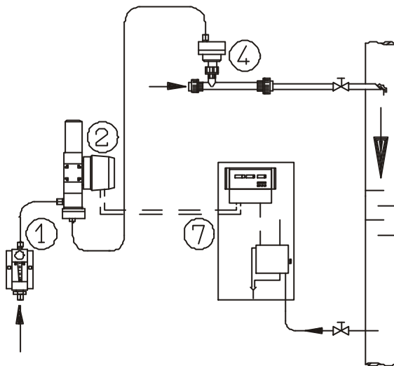
Circuit de régulation fermé
